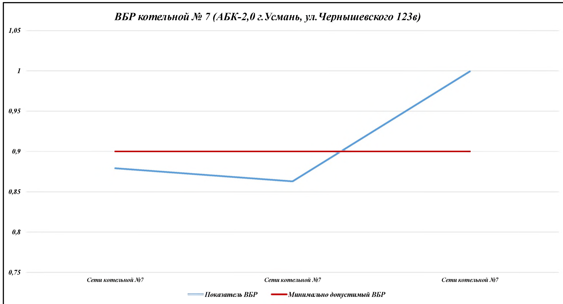
Рисунок 11.3.6 – ВБР котельной № 7 (АБК-2,0 г. Усмань, ул. Чернышевского, д. 123в)
