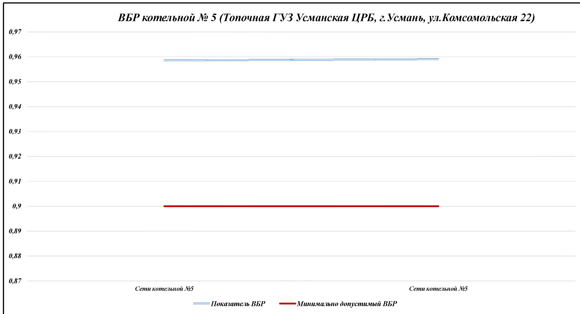
Рисунок 11.3.4 – ВБР котельной № 5 (Топочная ГУЗ Усманская ЦРБ, г. Усмань, ул. Комсомольская, д. 22)
