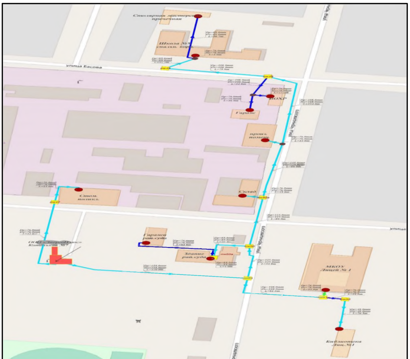
Рисунок 3.5.3 – Цветовое отображение уд. лин. потерь после моделирования
