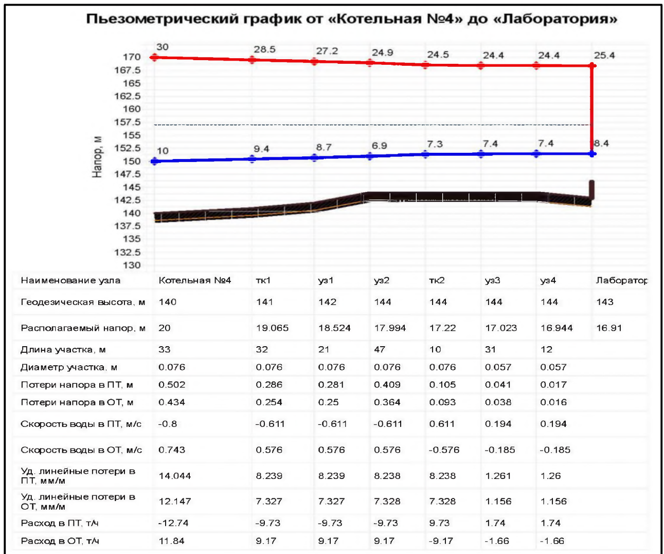
Рисунок 1.3.8.2 – Пьезометрический график Котельной № 4 (ГУЗ «Усманский противотуберкулезный детский санаторий»)
