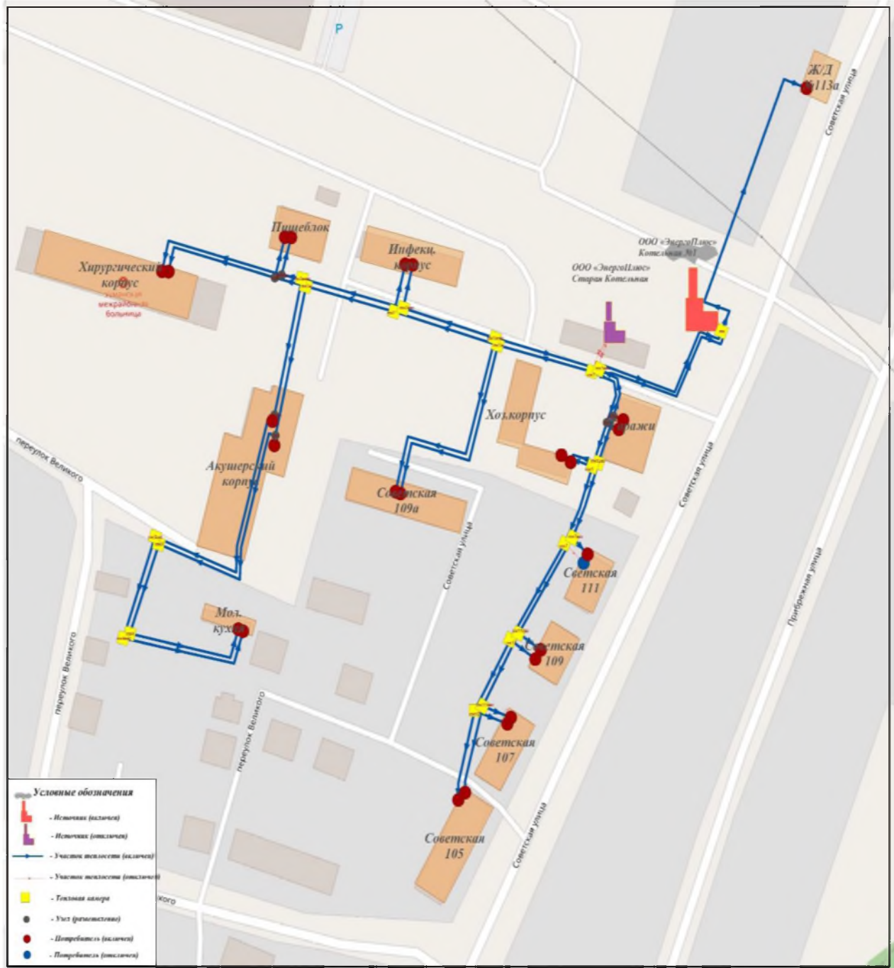
Рисунок 3.1.1 – Графическое представление объектов системы теплоснабжения Котельной №2
