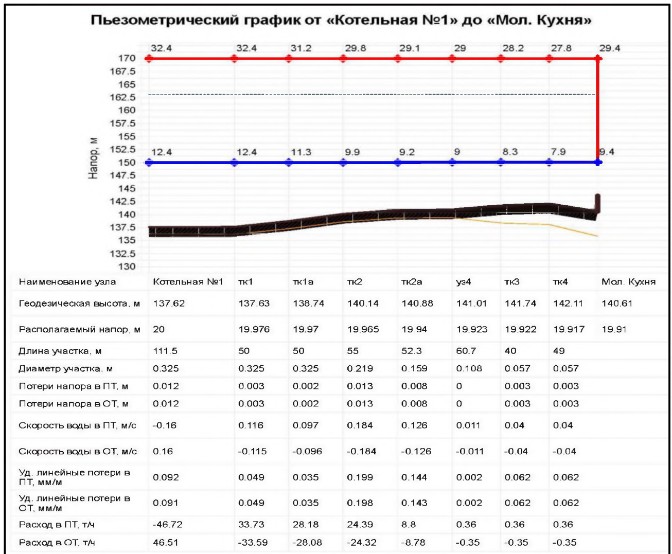
Рисунок 1.3.8.1 – Пьезометрический график Котельная №1 (Старая котельная ГУЗ Усманская ЦРБ, г. Усмань, ул. К. Маркса, д. 118)
