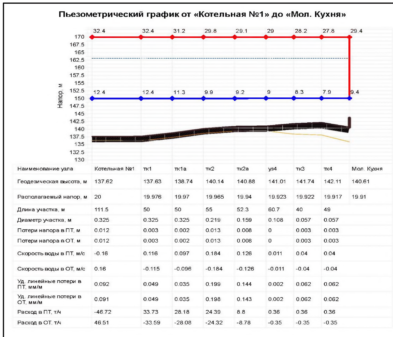
Рисунок 3.1.1.1 – Гидравлическая модель системы теплоснабжения
