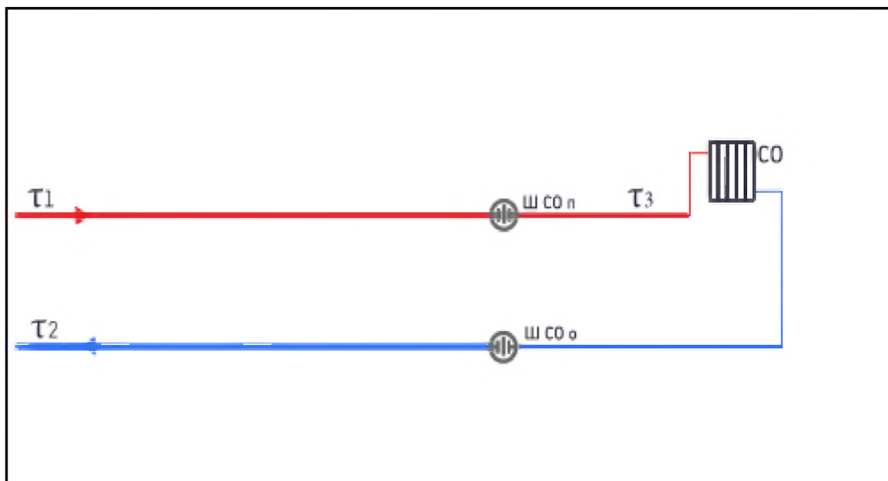
Рисунок 1.3.16.1 – Принципиальная тепловая схема присоединения потребителей городского поселения город Усмань «Потребитель с непосредственным присоединением СО»
