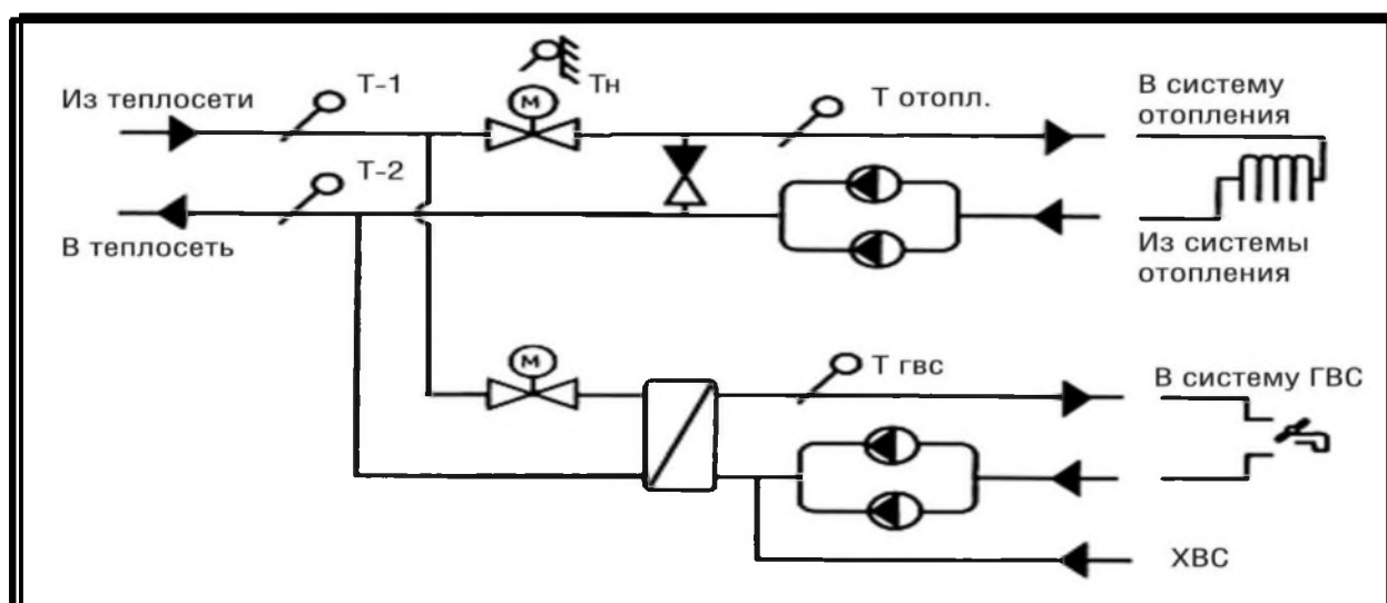
Рисунок 9.1.1. Присоединение ГВС по одноступенчатой схеме при зависимой схеме подключения системы отопления
