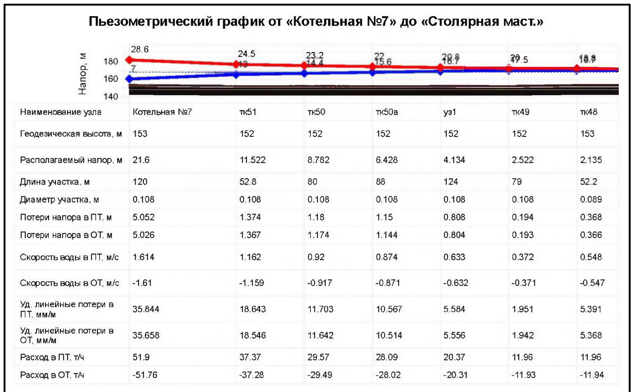
Рисунок 1.3.8.5 – Пьезометрический график Котельной №7(АБК-2,0 г. Усмань, ул. Чернышевского, д. 123в)
