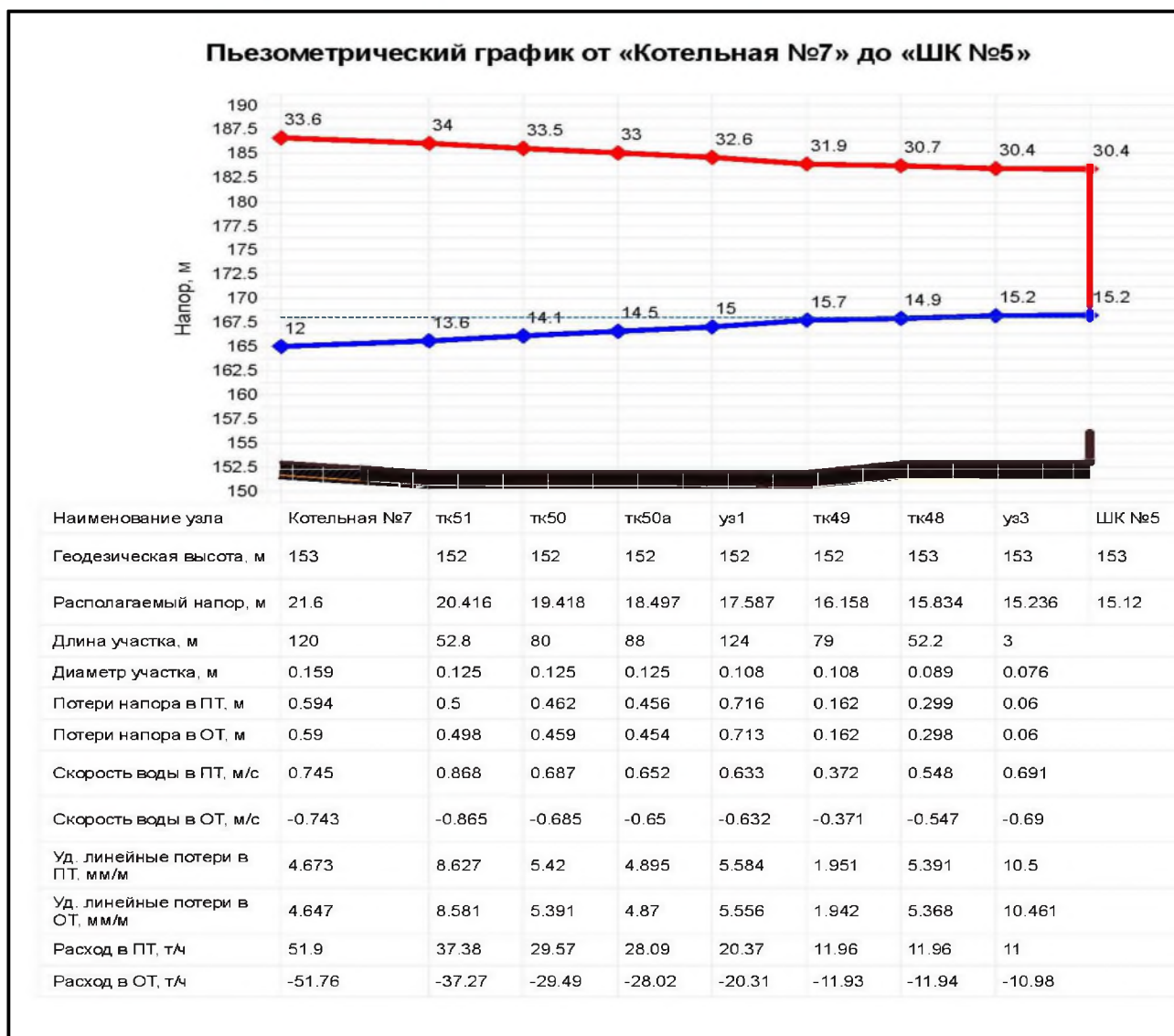
Рисунок 1.6.3.2 – Пьезометрический график Котельной №7(АБК-2,0 г. Усмань, ул. Чернышевского, д. 123в) (увеличение диаметра)
