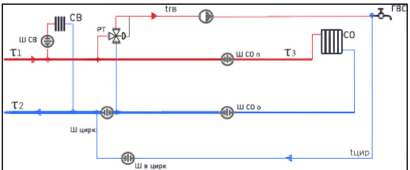
Рисунок 1.3.16.3 – Принципиальная тепловая схема присоединения потребителей городского поселения город Усмань «Потребитель с открытым водоразбором на ГВС и непосредственным присоединением СО»
