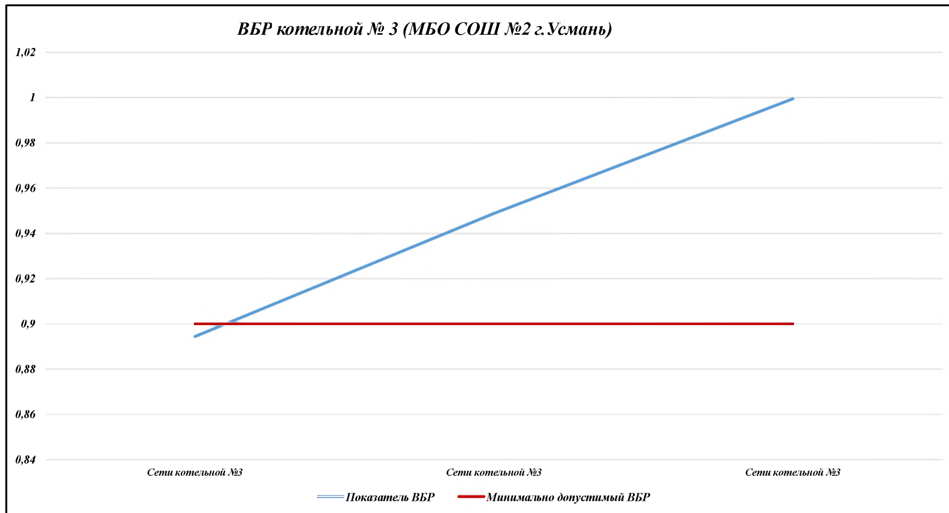
Рисунок 11.3.2 – ВБР котельной № 3 (МБОУ СОШ №2 г. Усмань)
