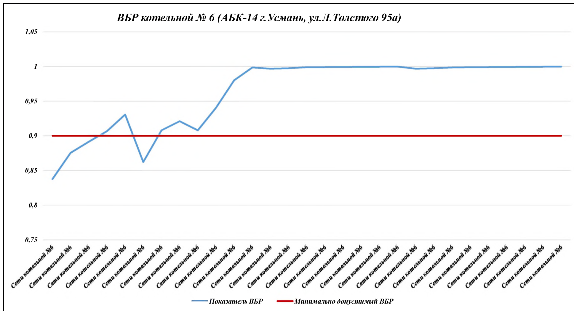
Рисунок 11.3.5 – ВБР котельной № 6 (АБК-14 г. Усмань, ул. Л. Толстого, д. 95а)
