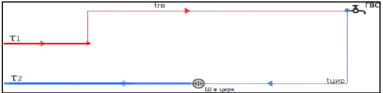
Рисунок 1.3.16.2 – Принципиальная тепловая схема присоединения потребителей городского поселения город Усмань «Потребитель с открытым водоразбором и циркуляционной линией»
