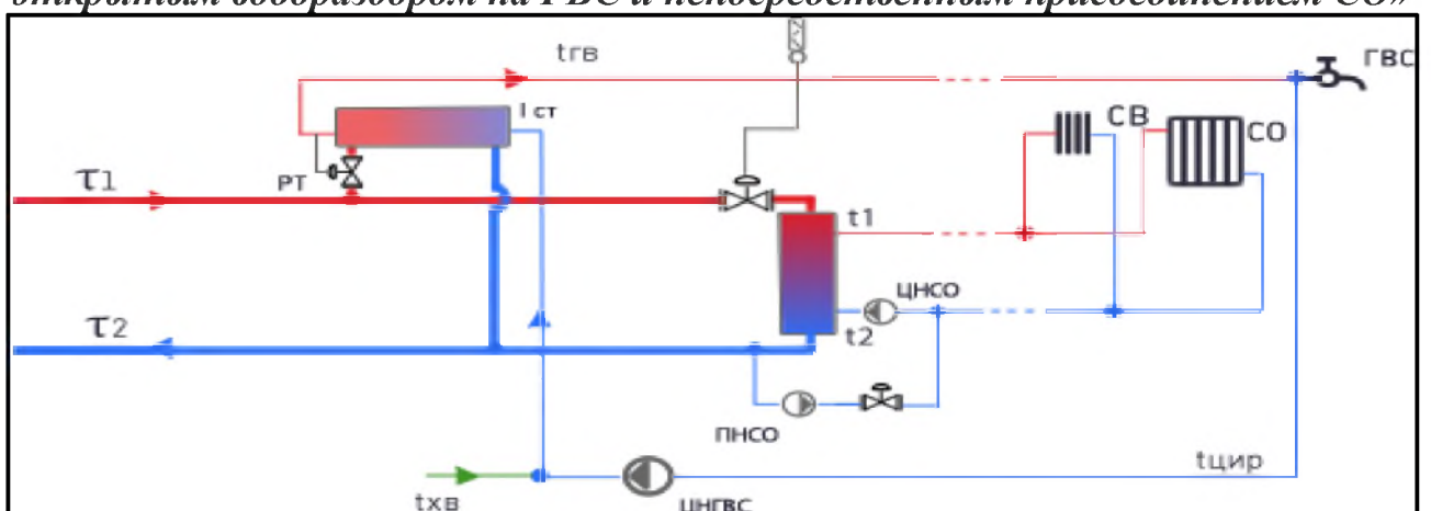
Рисунок 1.3.16.4 – Принципиальная тепловая схема присоединения потребителей городского поселения город Усмань «ЦТП с параллельным подключением подогревателей ГВС и независимым присоединением СО и СВ»
