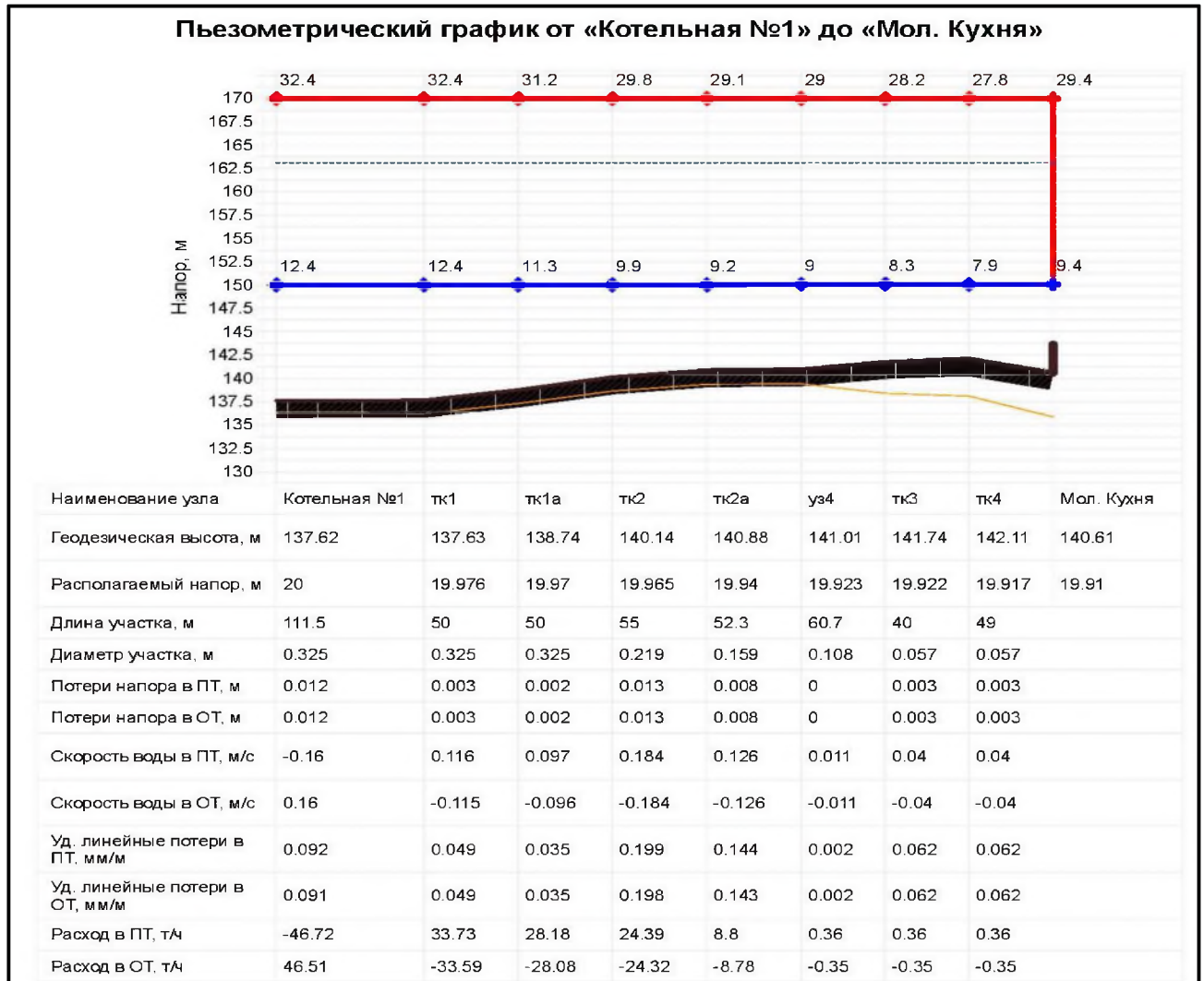
Рисунок 3.10.1 – Пьезометрический график
